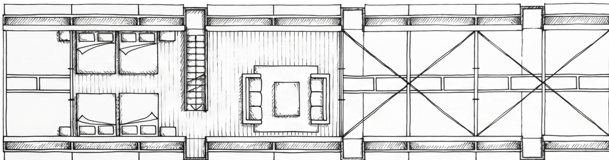
Planta altillo
